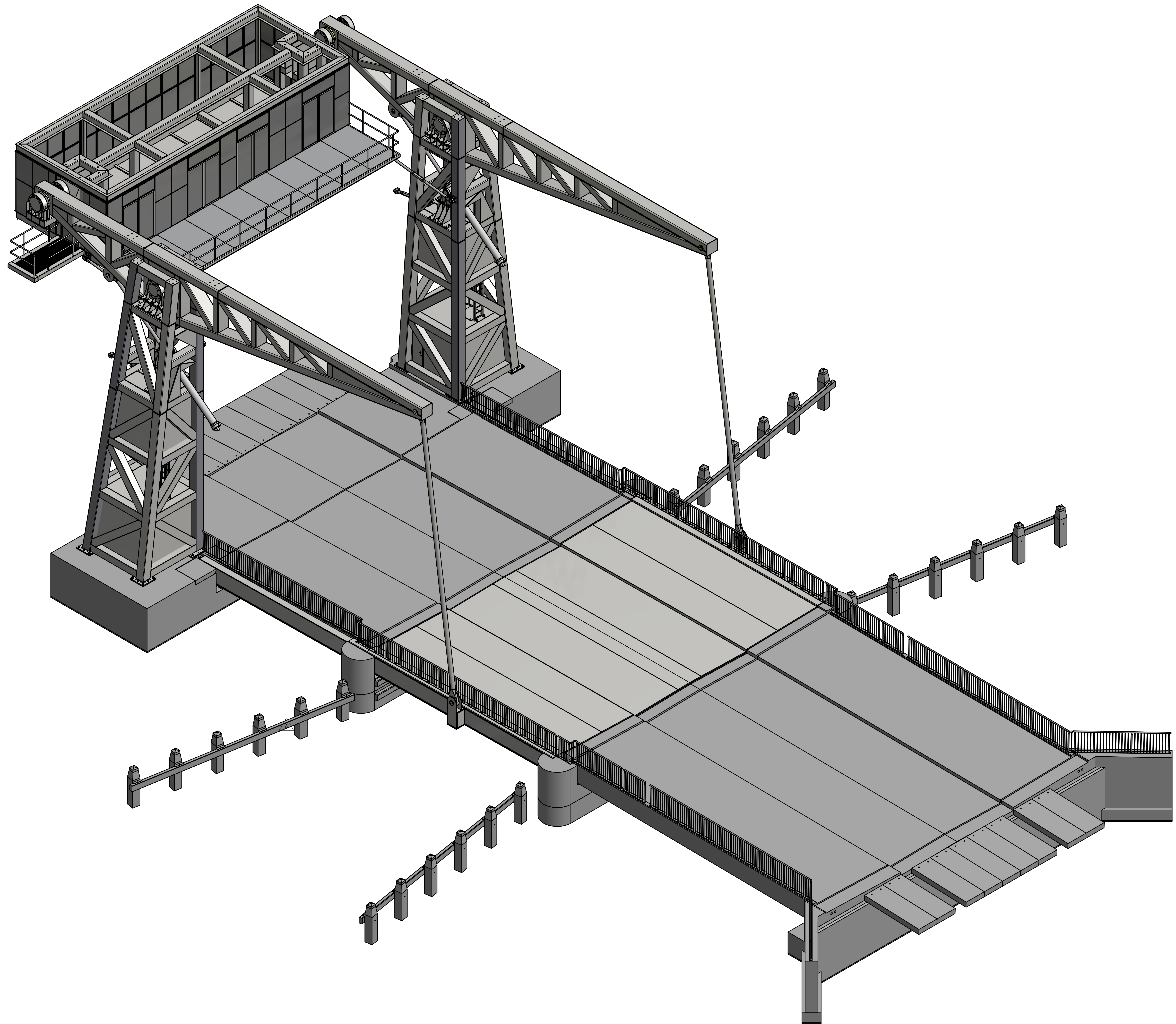
brug-gesloten ( 1 : 50 )
