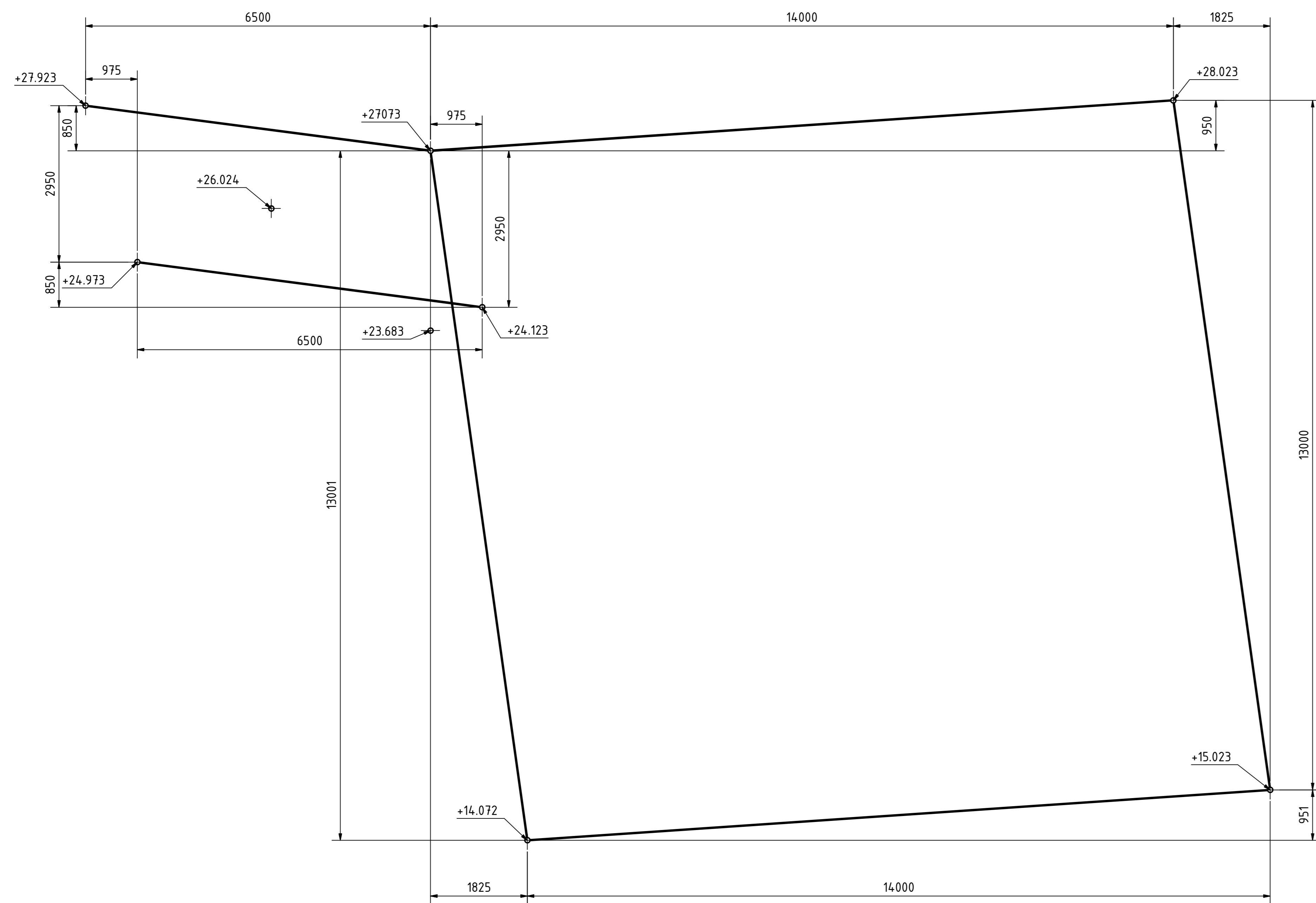
systemlijn(en) ( 1 : 50 )
