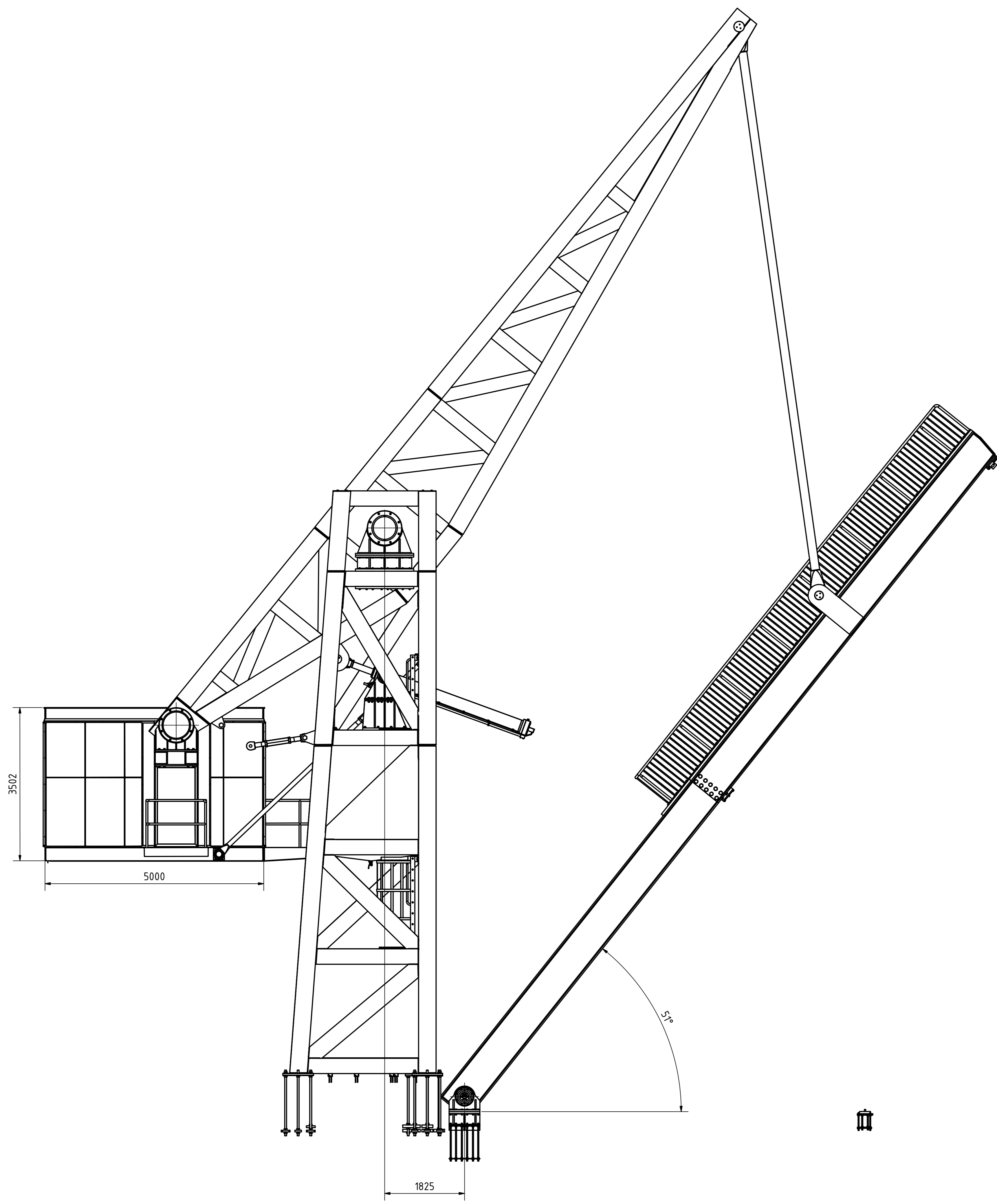
voor-aanzicht ( 1 : 50 )
