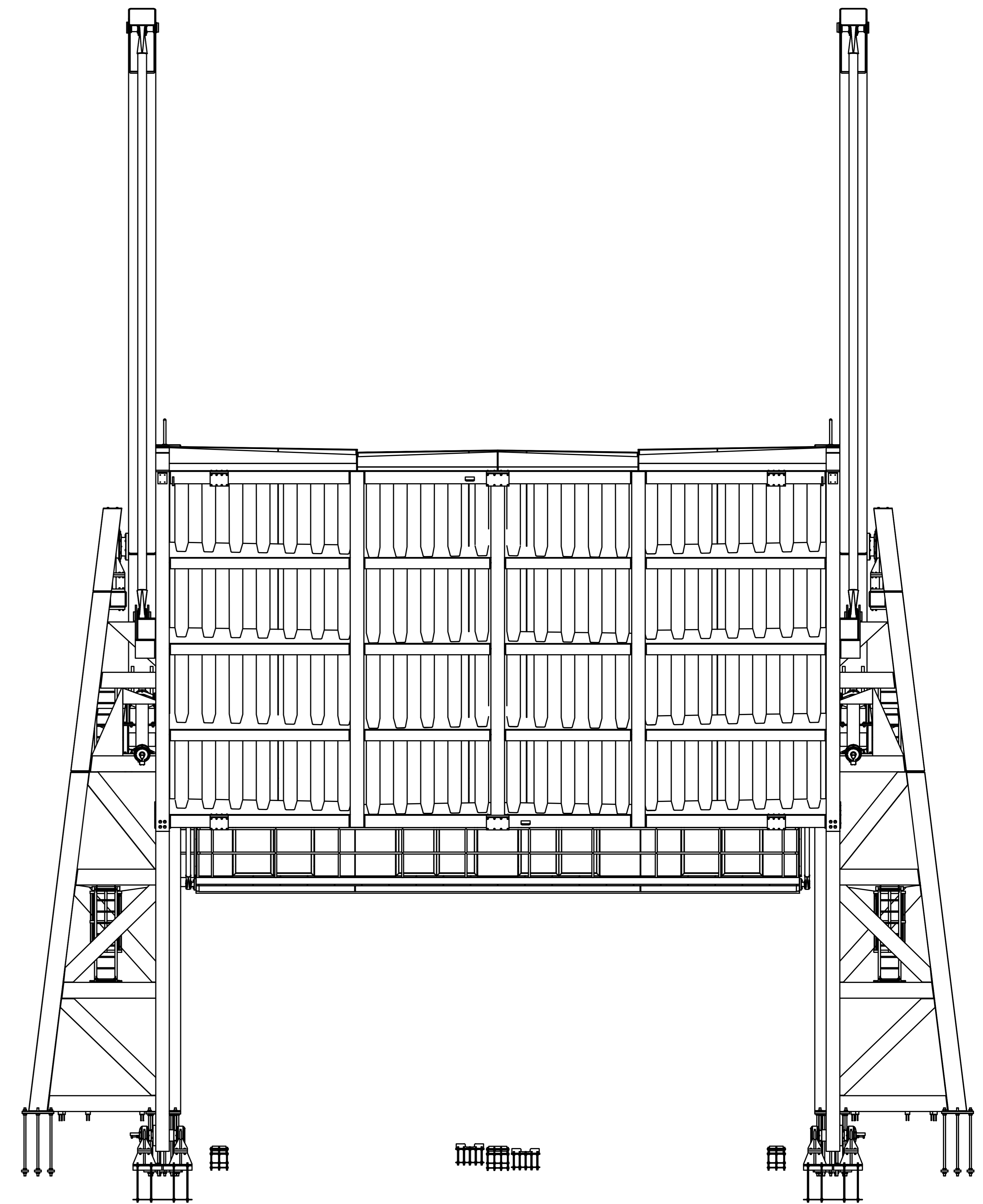
zij-aanzicht ( 1 : 50 )
