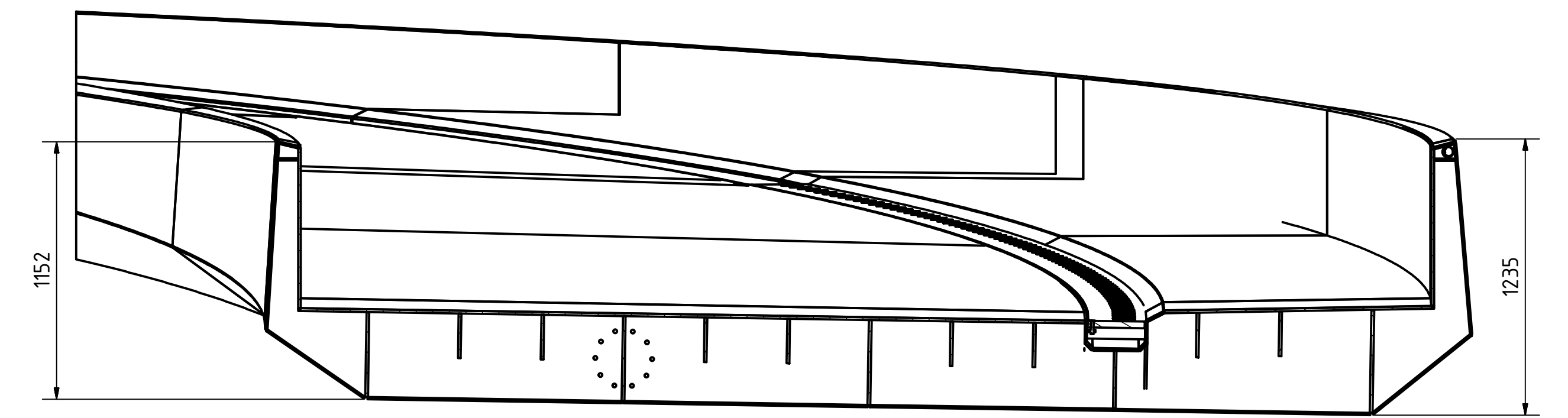
C-C ( 1 : 20 )
