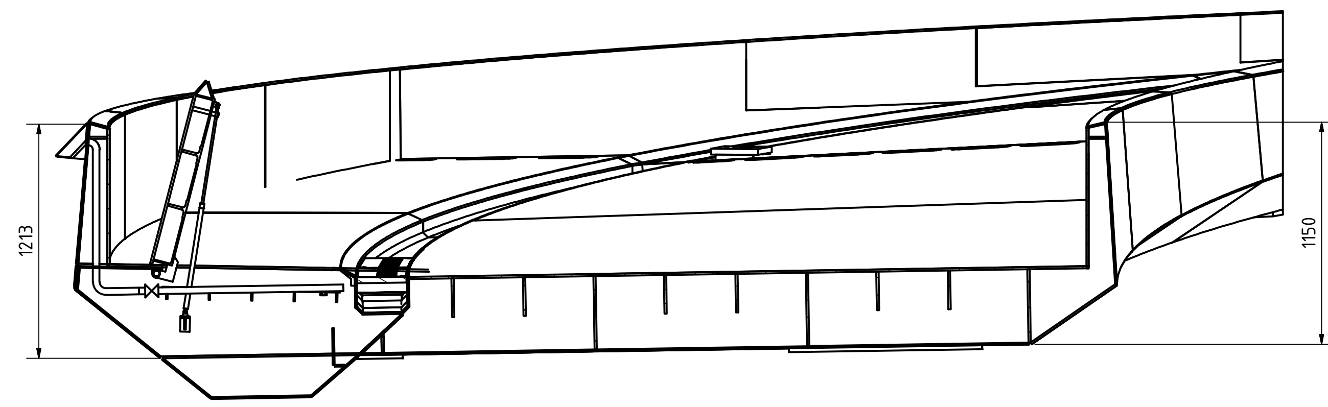
A-A ( 1 : 20 )
