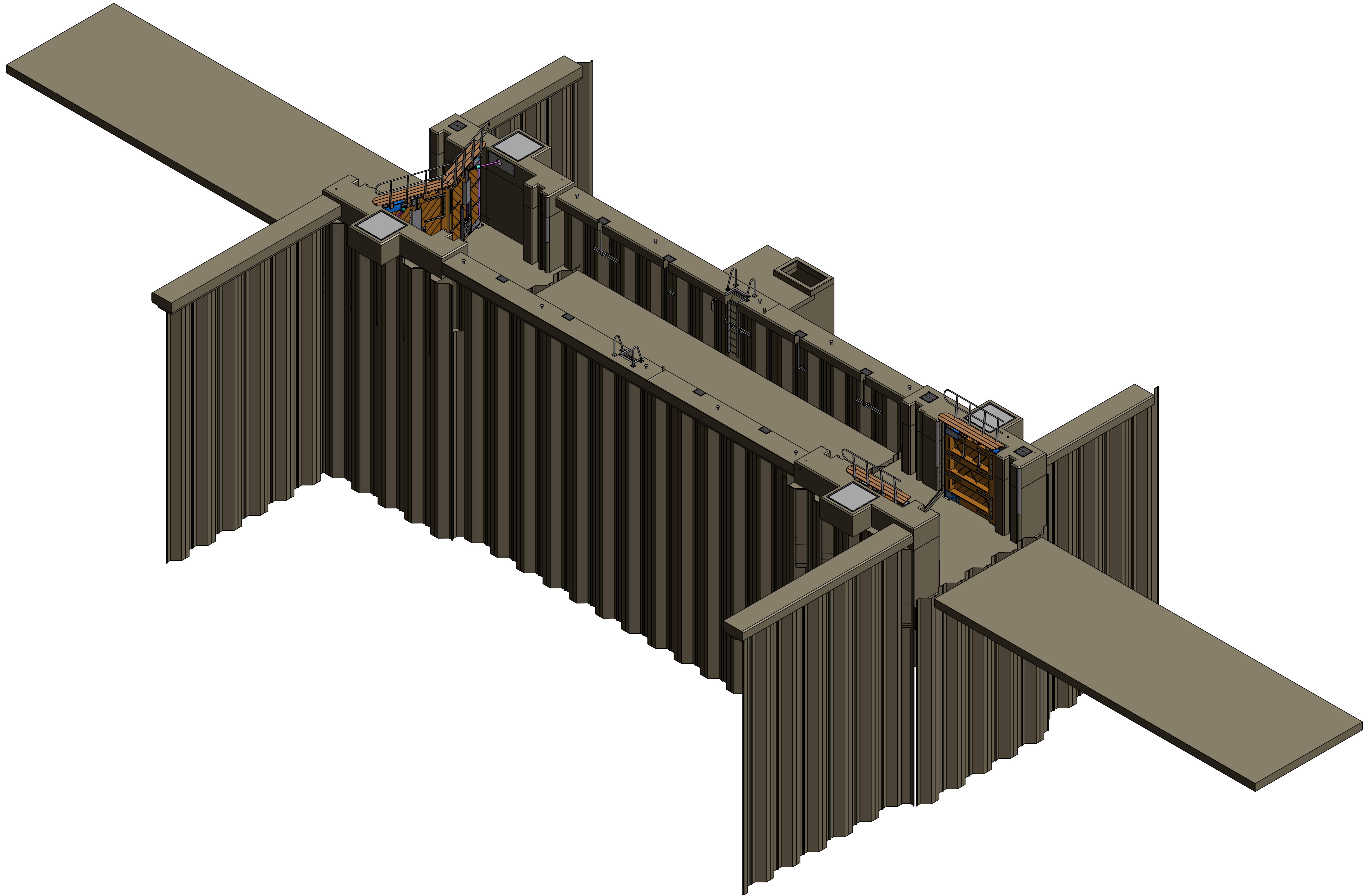
Overzicht ( 1 : 50 )
