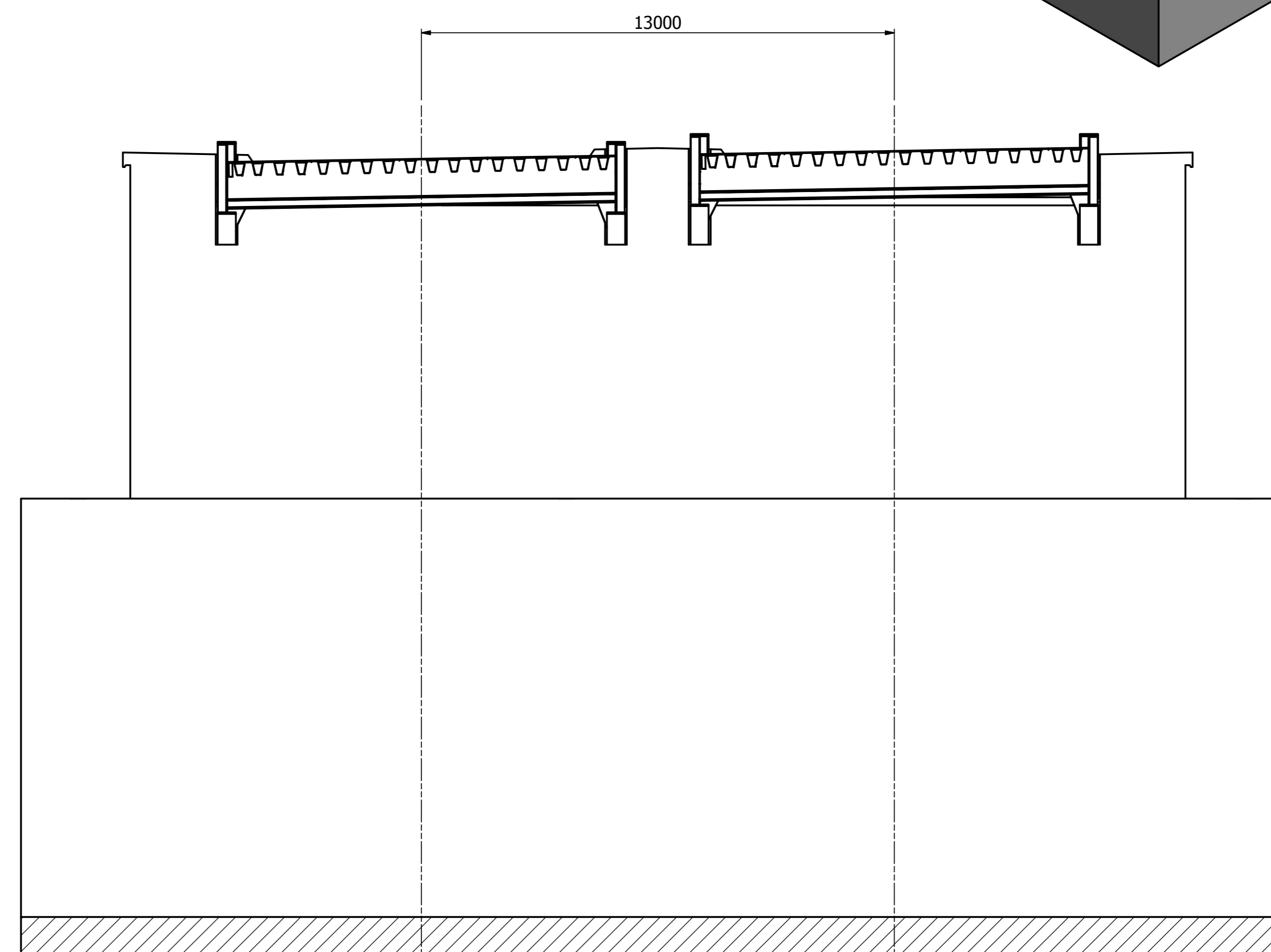
B-B ( 1 : 100 )
