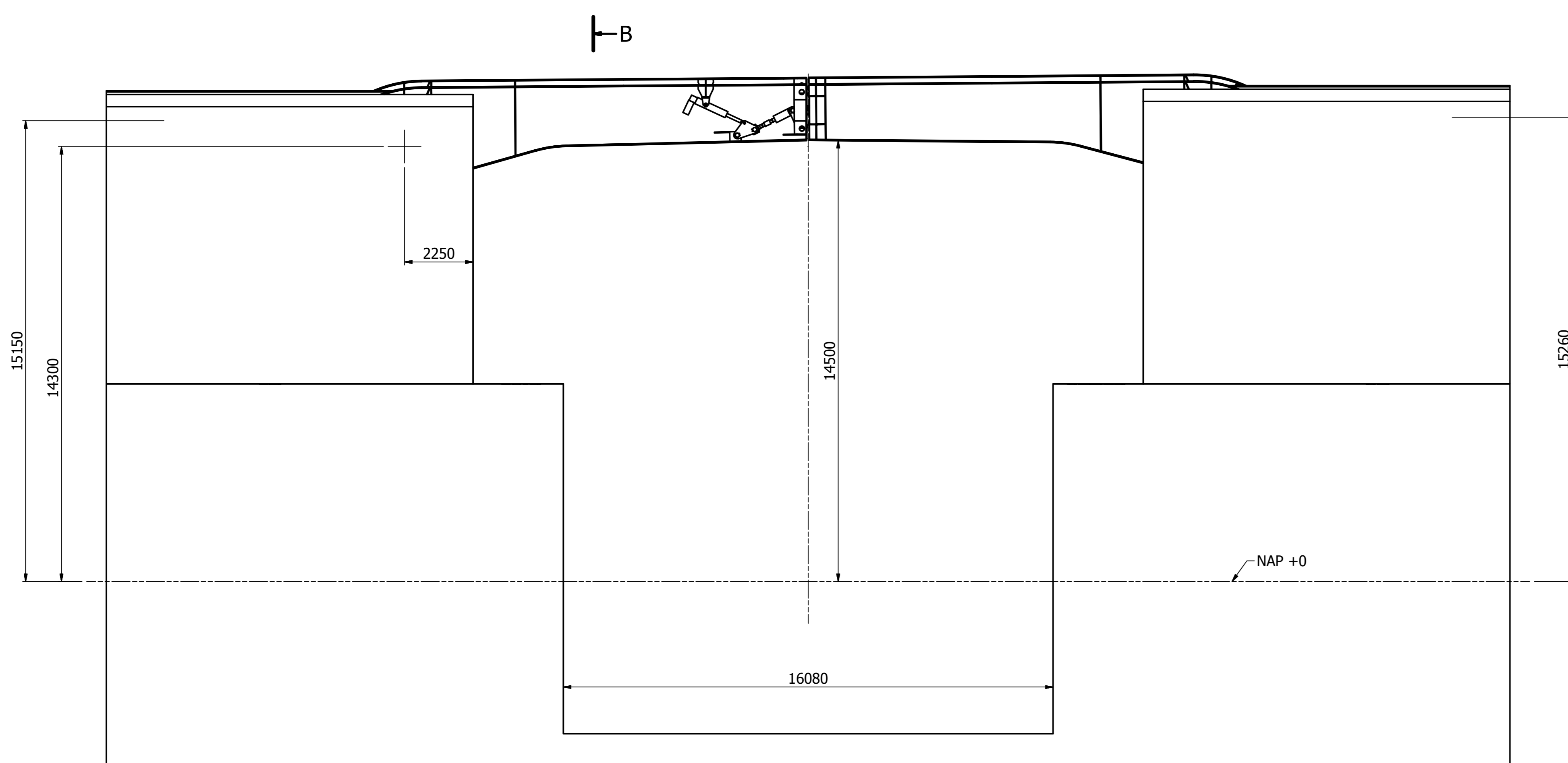
vooraanzicht ( 1 : 100 )
