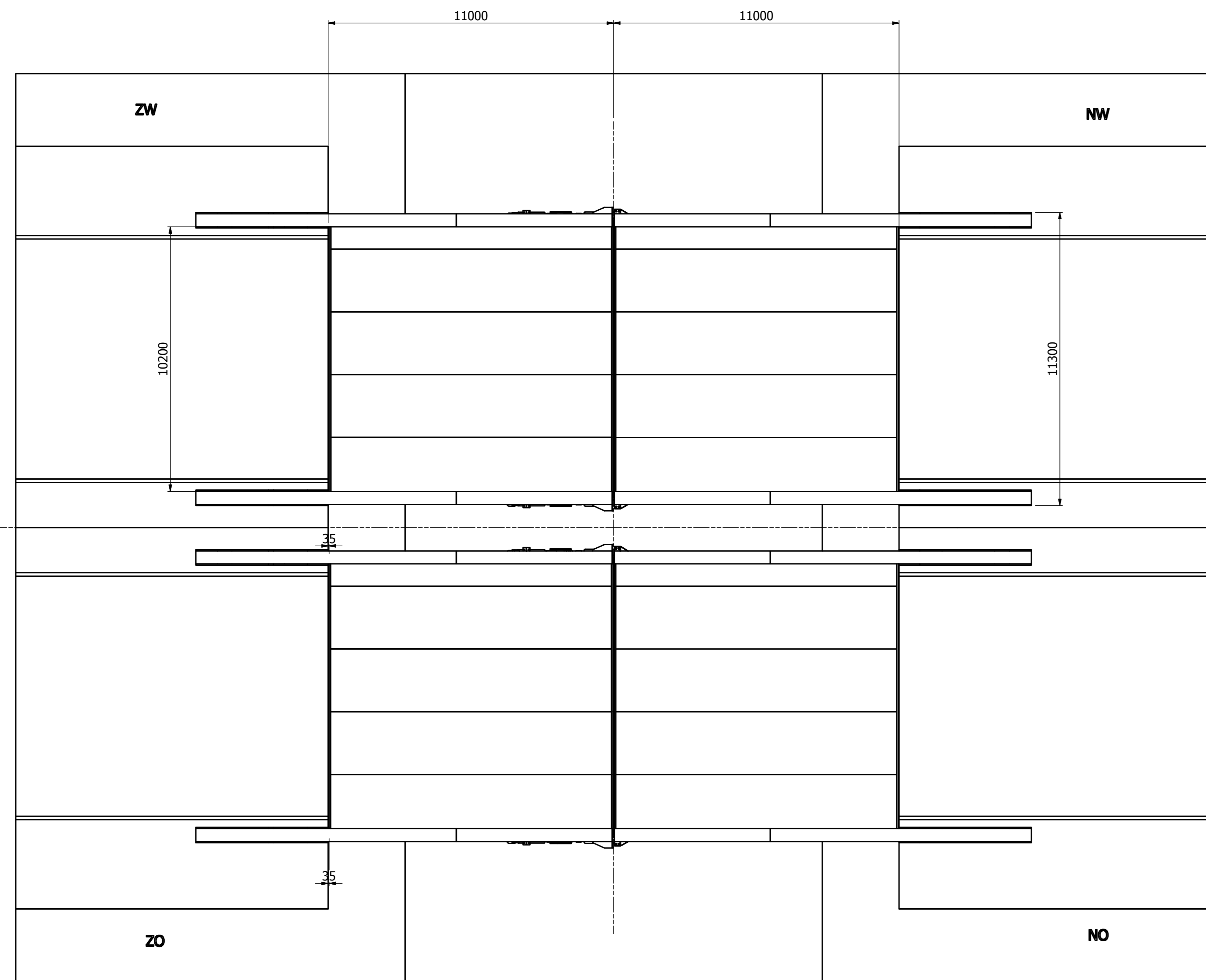
bovenaanzicht ( 1 : 100 )
