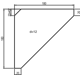
schetsplaat (1 : 2)
