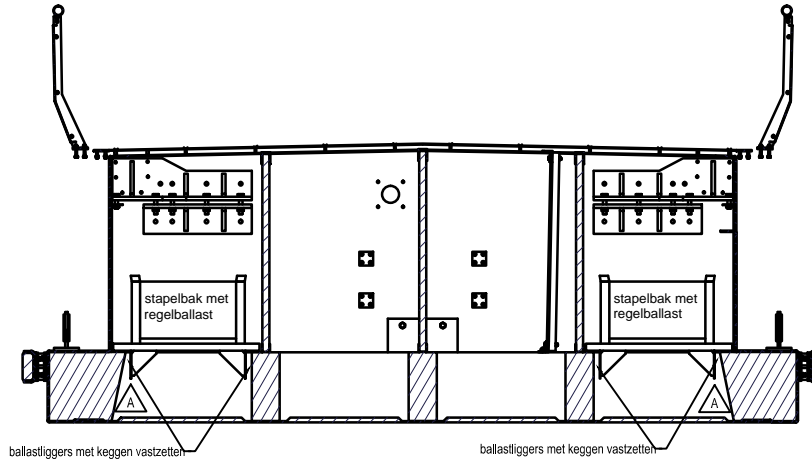
A-A (1 : 20)
