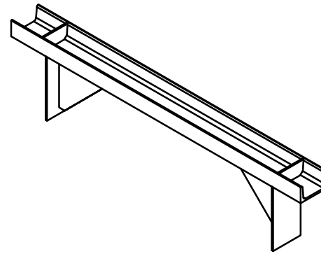
samengestelde ligger (1 : 5)
