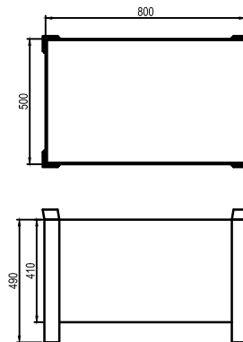
samengestelde ligger (1 : 5)
