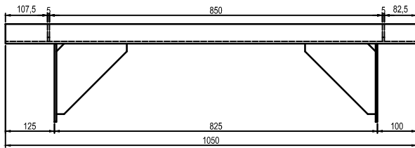
vooraanzicht (1 : 5)
