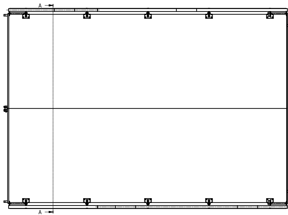
bovenaanzicht ( 1 : 20 )
