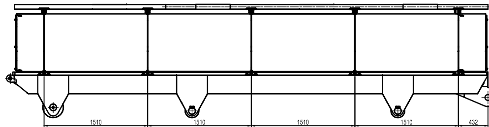
vooraanzicht ( 1 : 20 )
