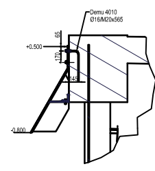
E (1 : 20)
