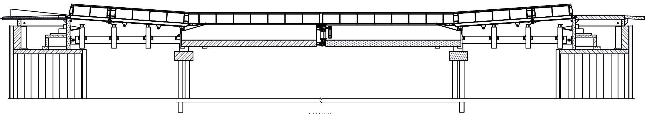
A-A ( 1 : 50 )
