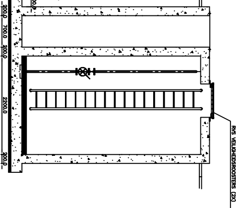
DOORSNIJDING C-C
